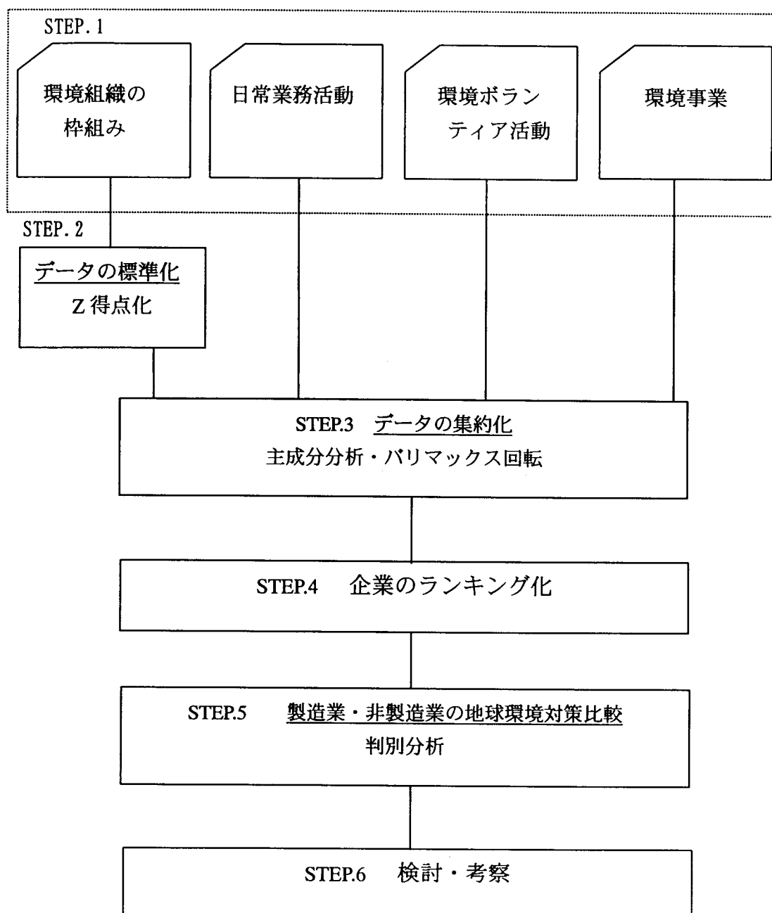
図 4-3-1 : 研究フロー
