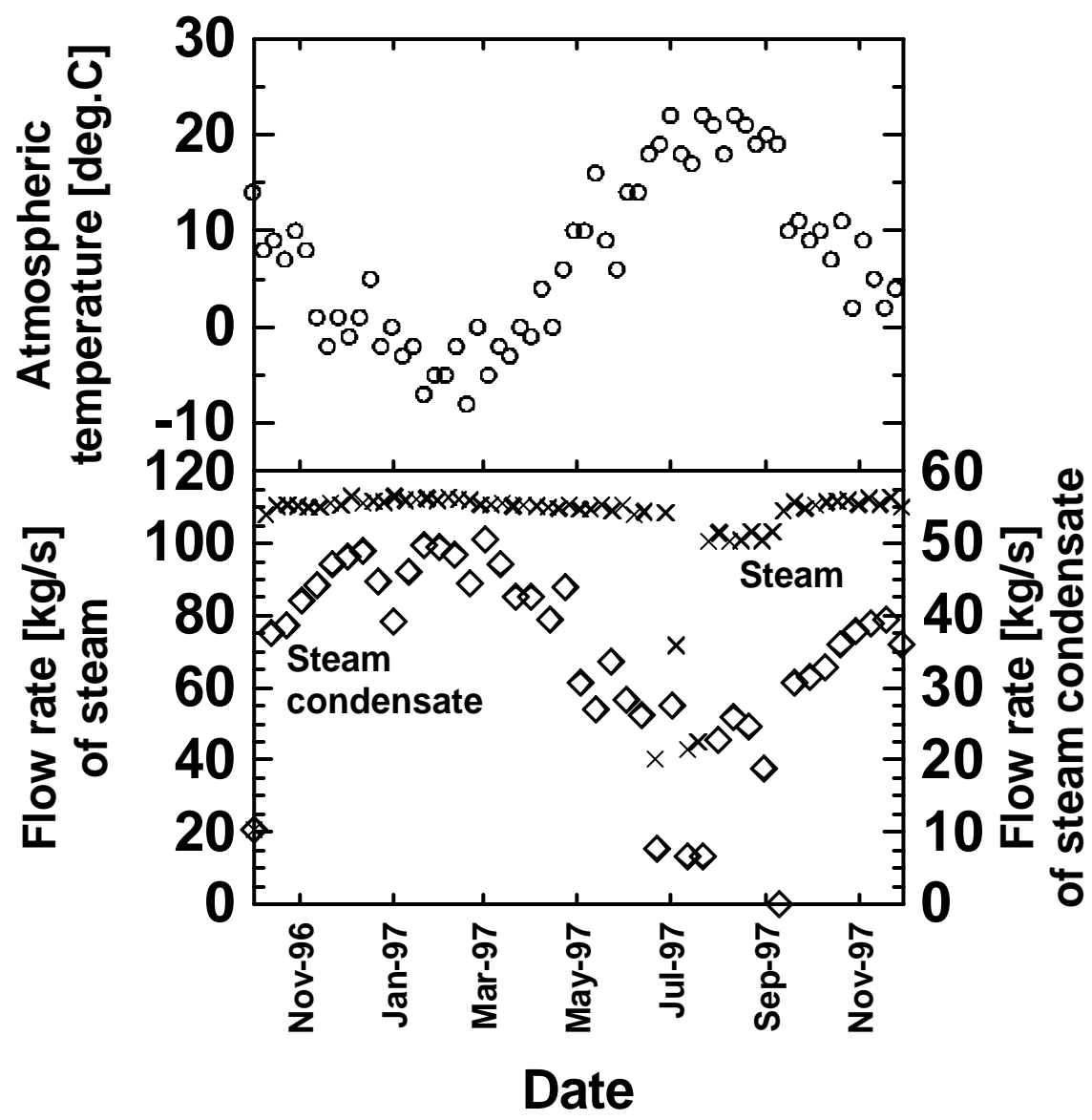
図4.5 総蒸気流量と蒸気復水還元流量、並びに気温の季節変動
