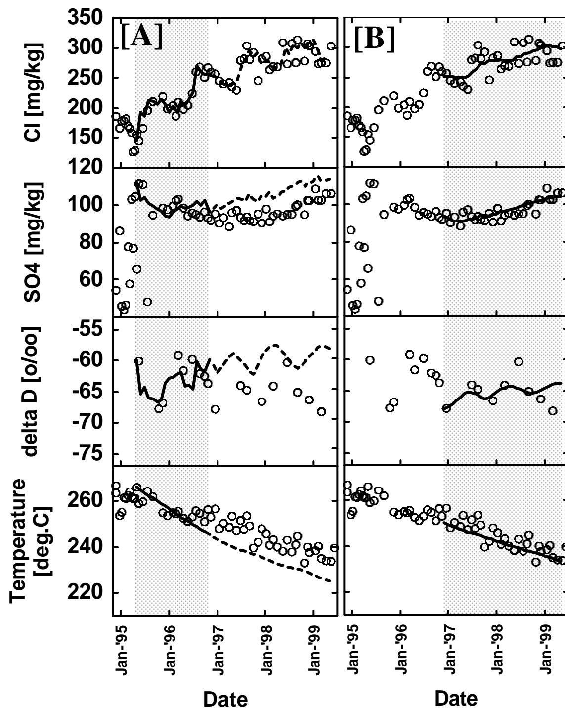
図4.10 実測値（○）計算結果（実線）とのマッチング（S-4坑）． [A]は解析期間の前半を、[B]はその後半を示す．
