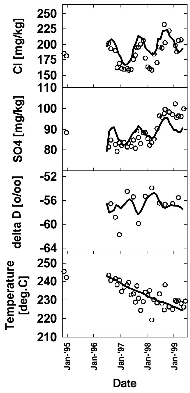
図4.8 実測値 ( ) 計算結果 (実線) とのマッチング (SB-1坑)
