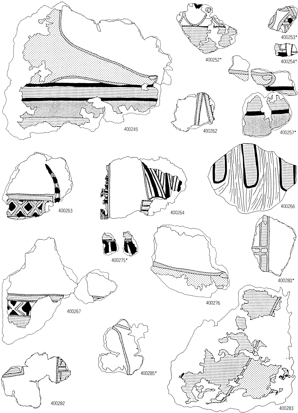
図 13 彩画片実測図(7) No.400245~400285 (縮尺:1/3. 但し 登録番号*は1/2)
