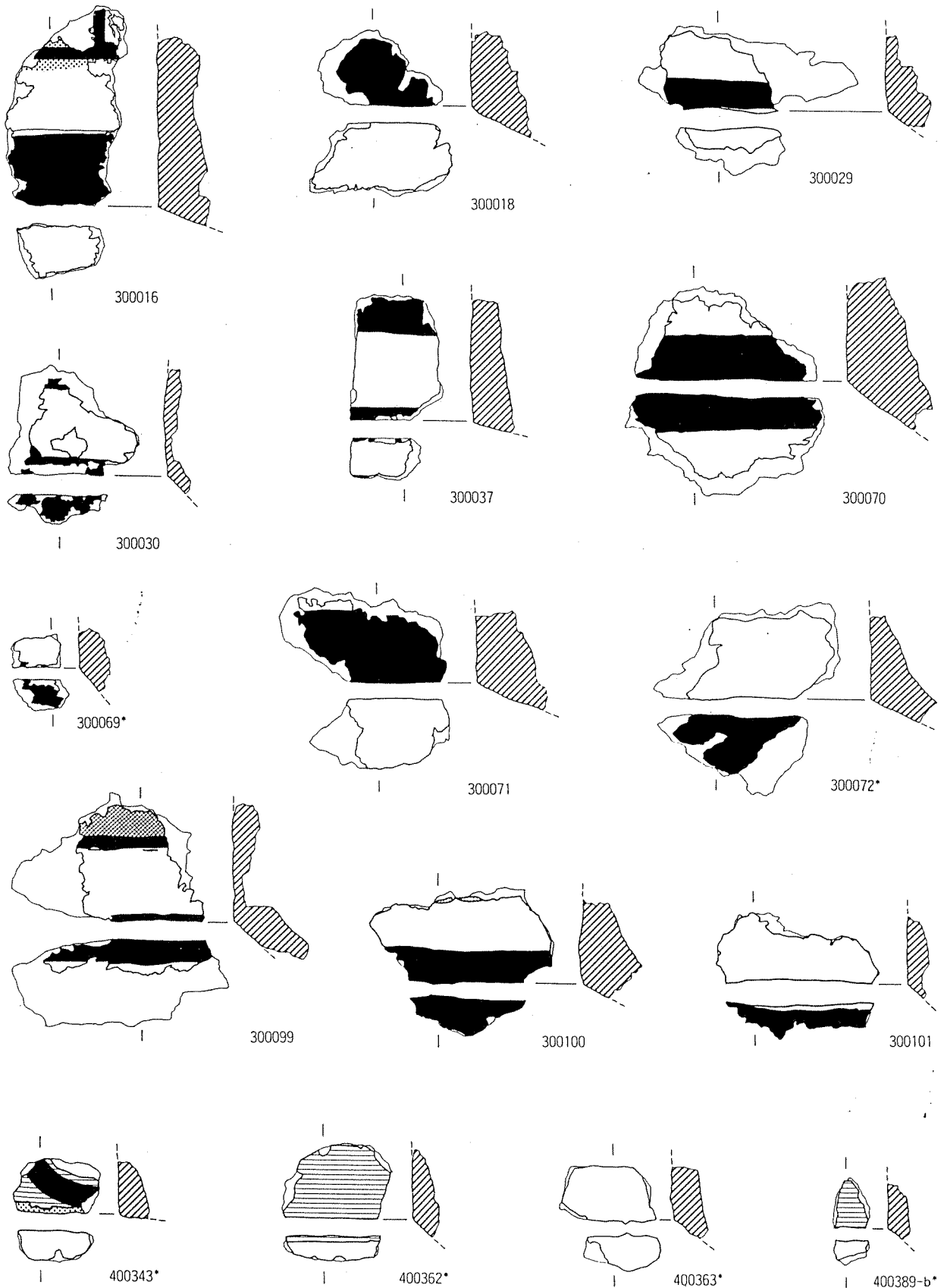
図 51 彩画片実測図・役物(1) コーナー
