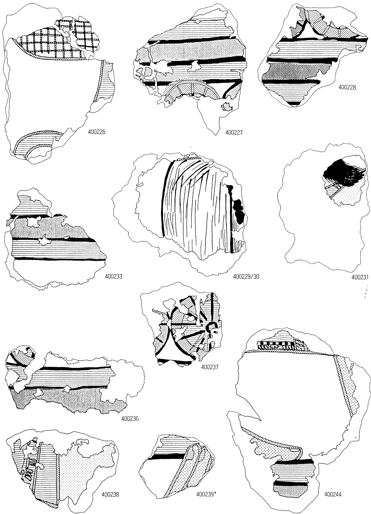
图 12 彩画片实测图(6) No.400226~400244
