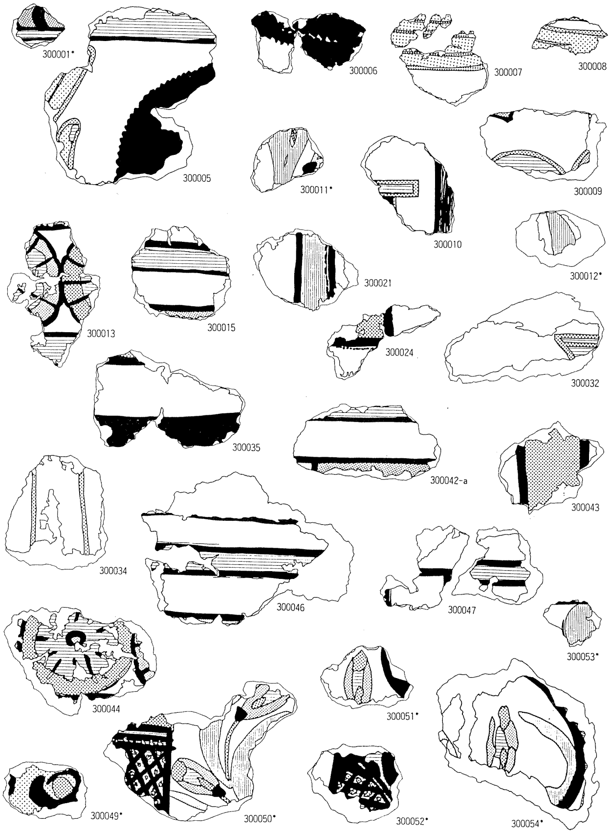
图 7 彩画片实测图(1) No.300001~300054
