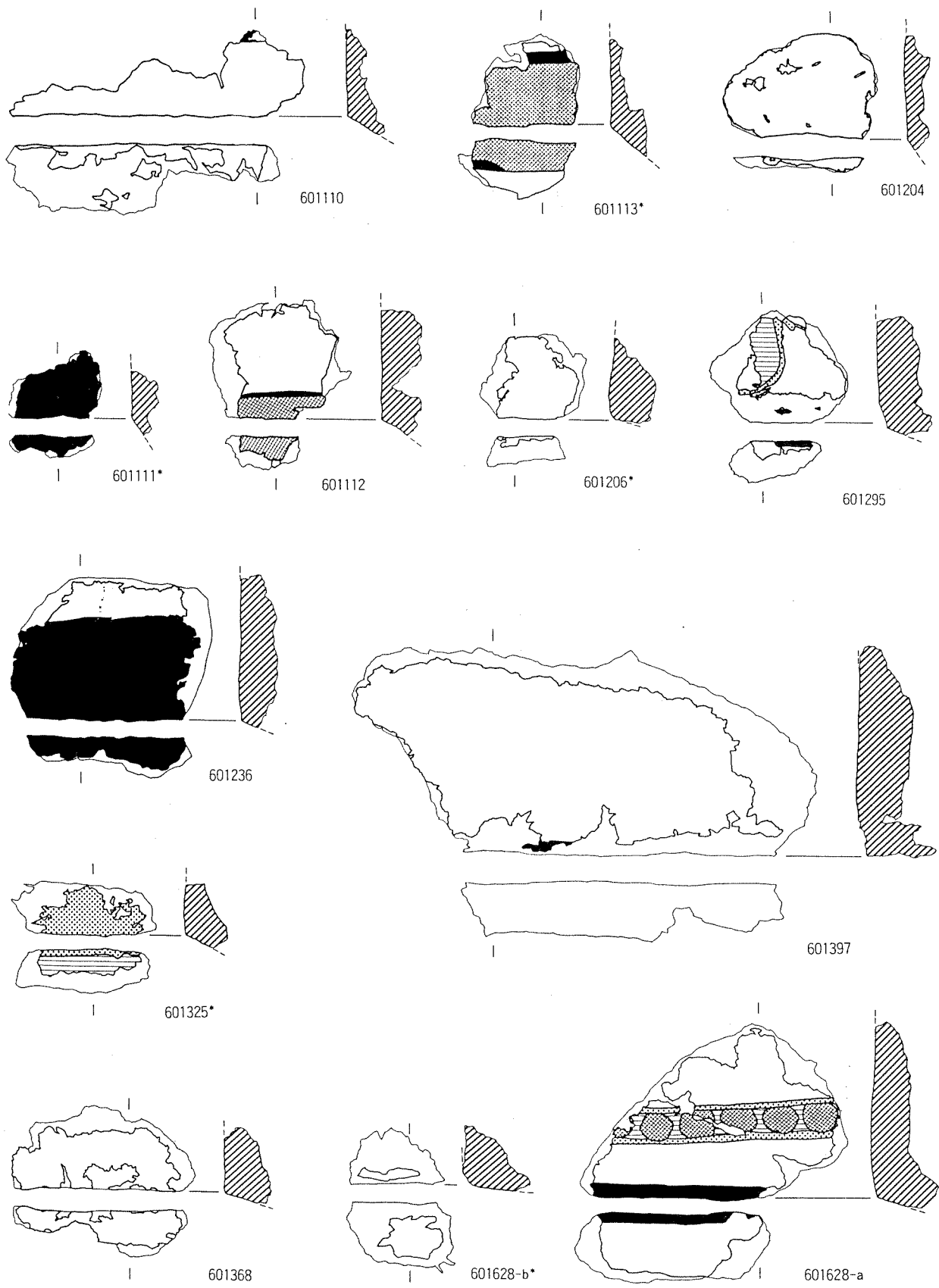
図 53 彩画片実測図・役物(3) コーナー
