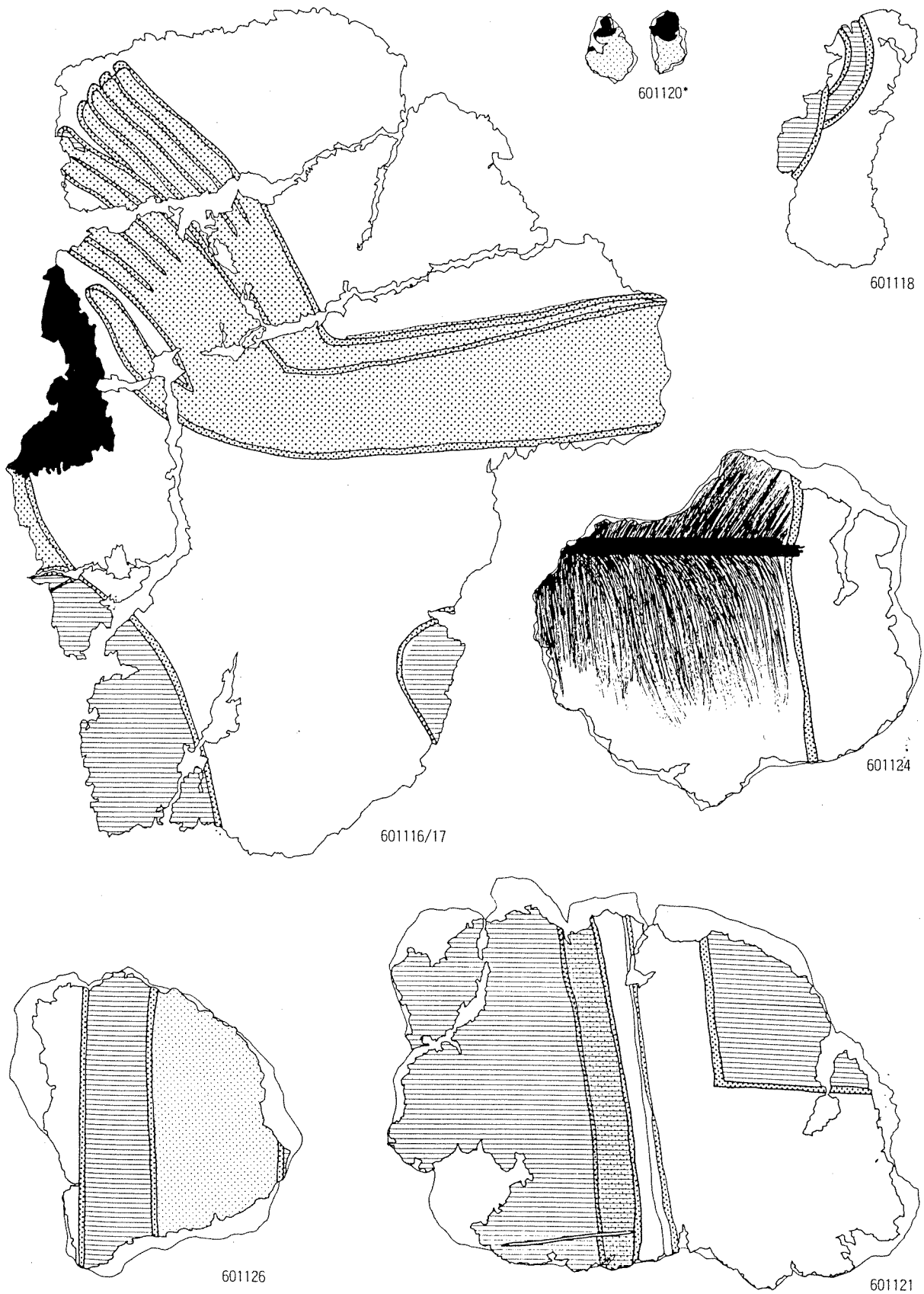
图 31 彩画片实测图(25) No.601116/17~601121,601124,601126
