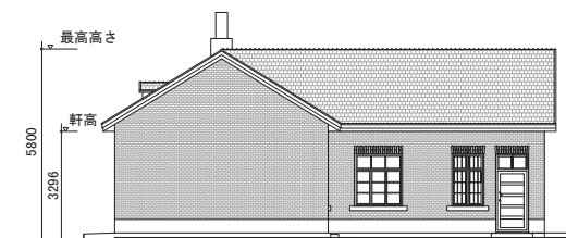
公共食堂東立面図
