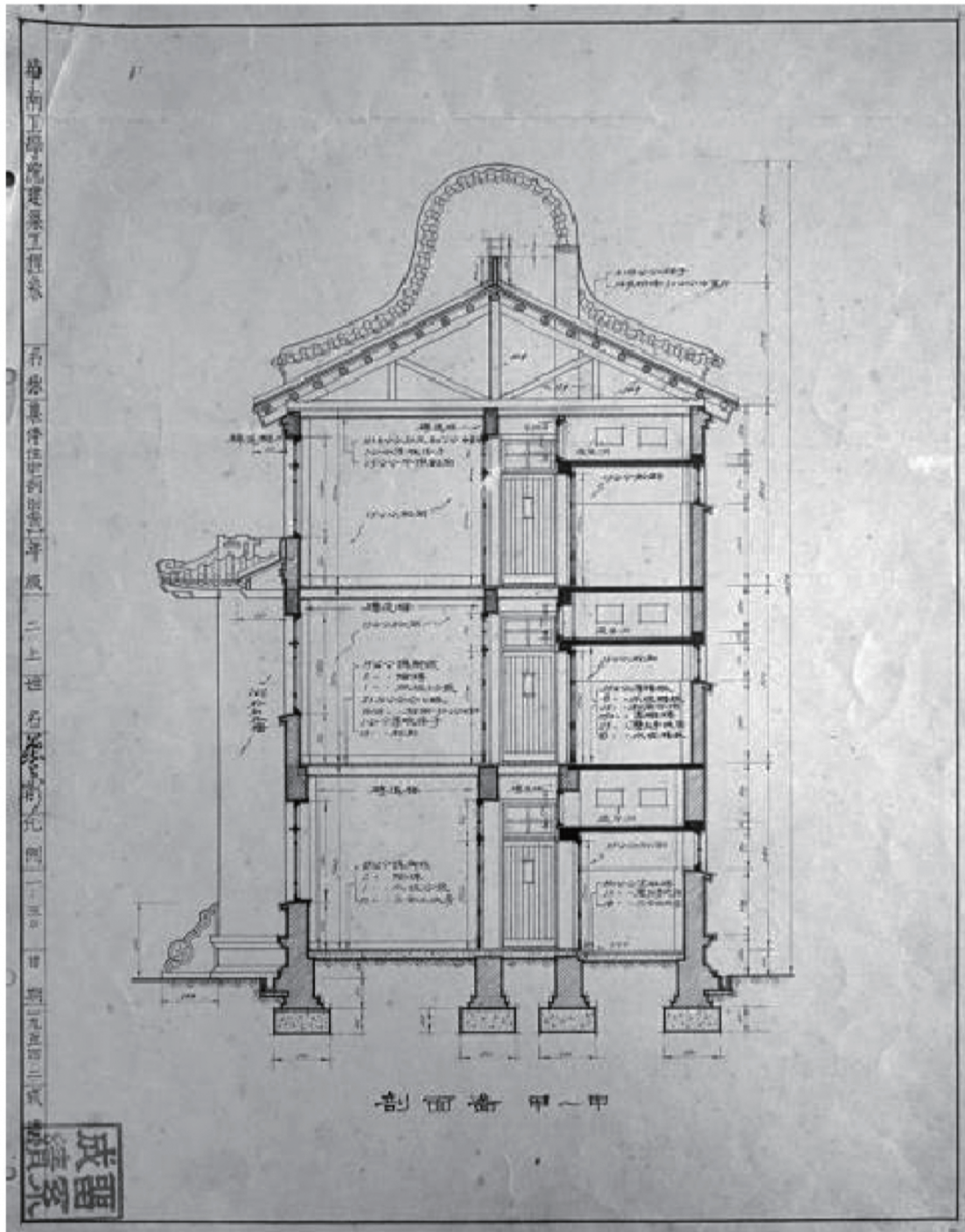
図3-4 華南工學院の学生によって設計された集団住宅断面図 注74)
