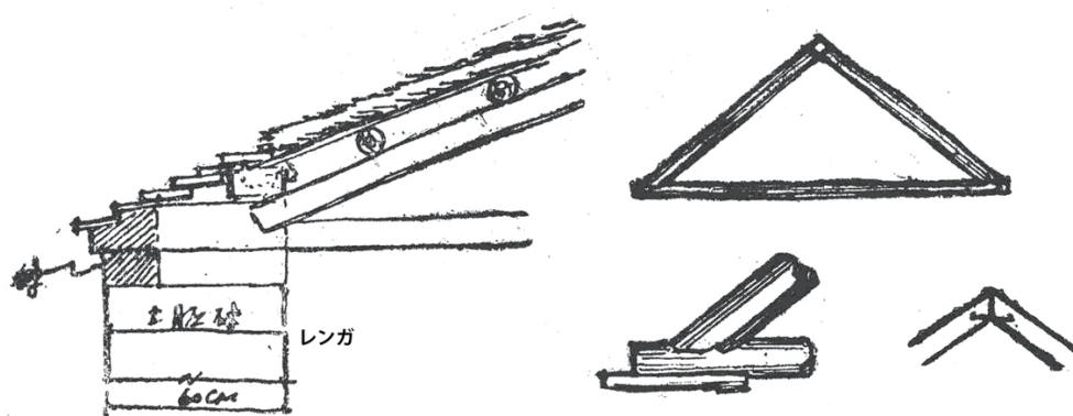
図5-6 衛星人民公社前湾村民家の屋根構造のスケッチ 注130)
