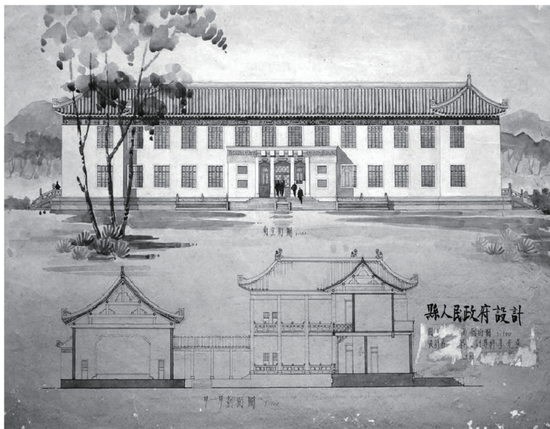
図3-3 華南工学院の学生によって設計された県人民政府図面, 1954 注73)
