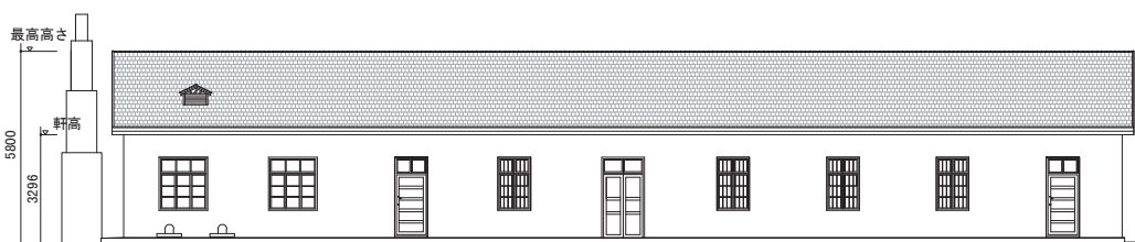
公共食堂南立面図
