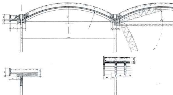
図3-11 屋根の細部構造, 輝く村落 注91)
