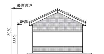
社員住居東立面図
