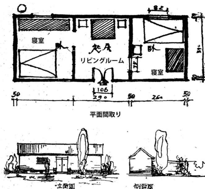
図4-5 前湾村の住宅平面間取りと立面図 注112)
