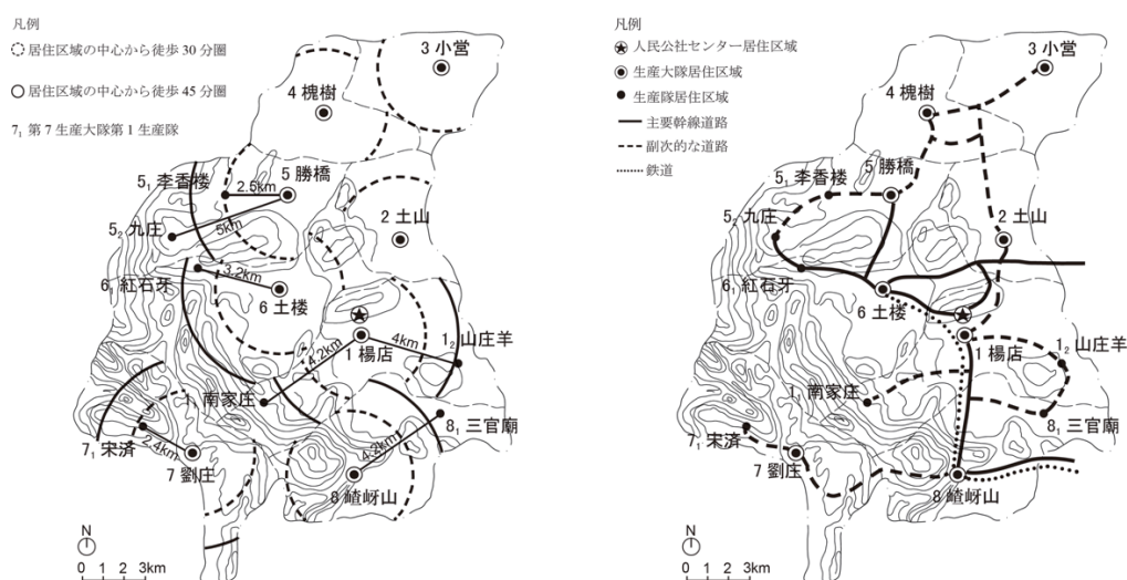
図2-8 衛星人民公社の生産隊居住区域の配置計画案と交通計画案 注48)
