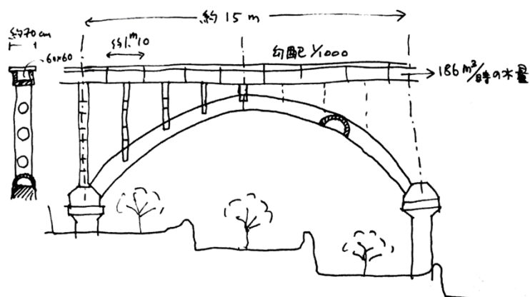
図 6-5 吉阪隆正による大沔人民公社の灌漑用水路のスケッチ 注159)
