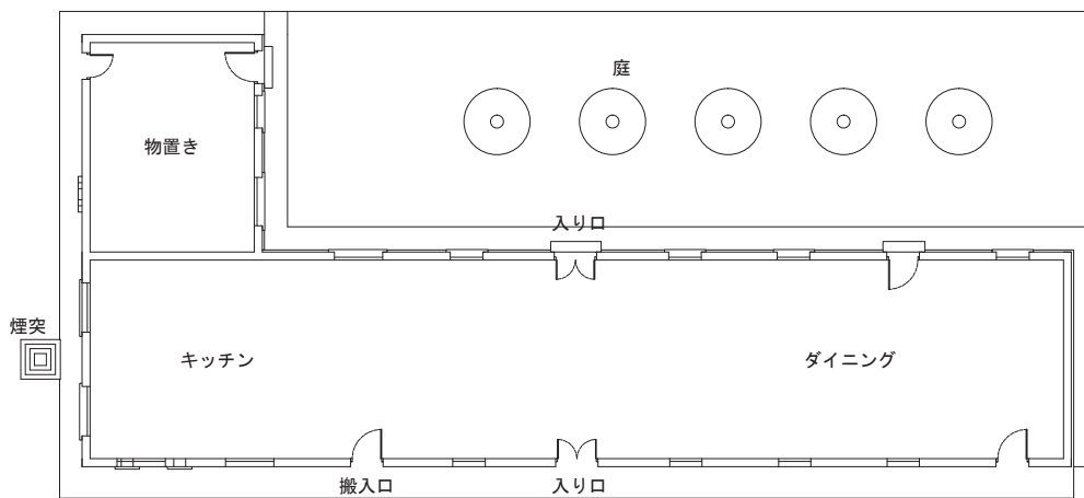
公共食堂一階平面図
