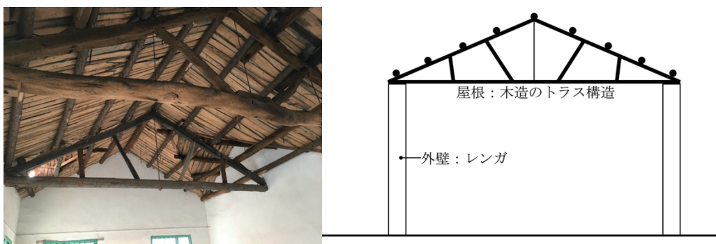
写真5-2 公共食堂の屋根の様子 図5-5 公共食堂の屋根構造のダイアグラム (筆者作成)
