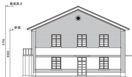
弁公楼東立面図
